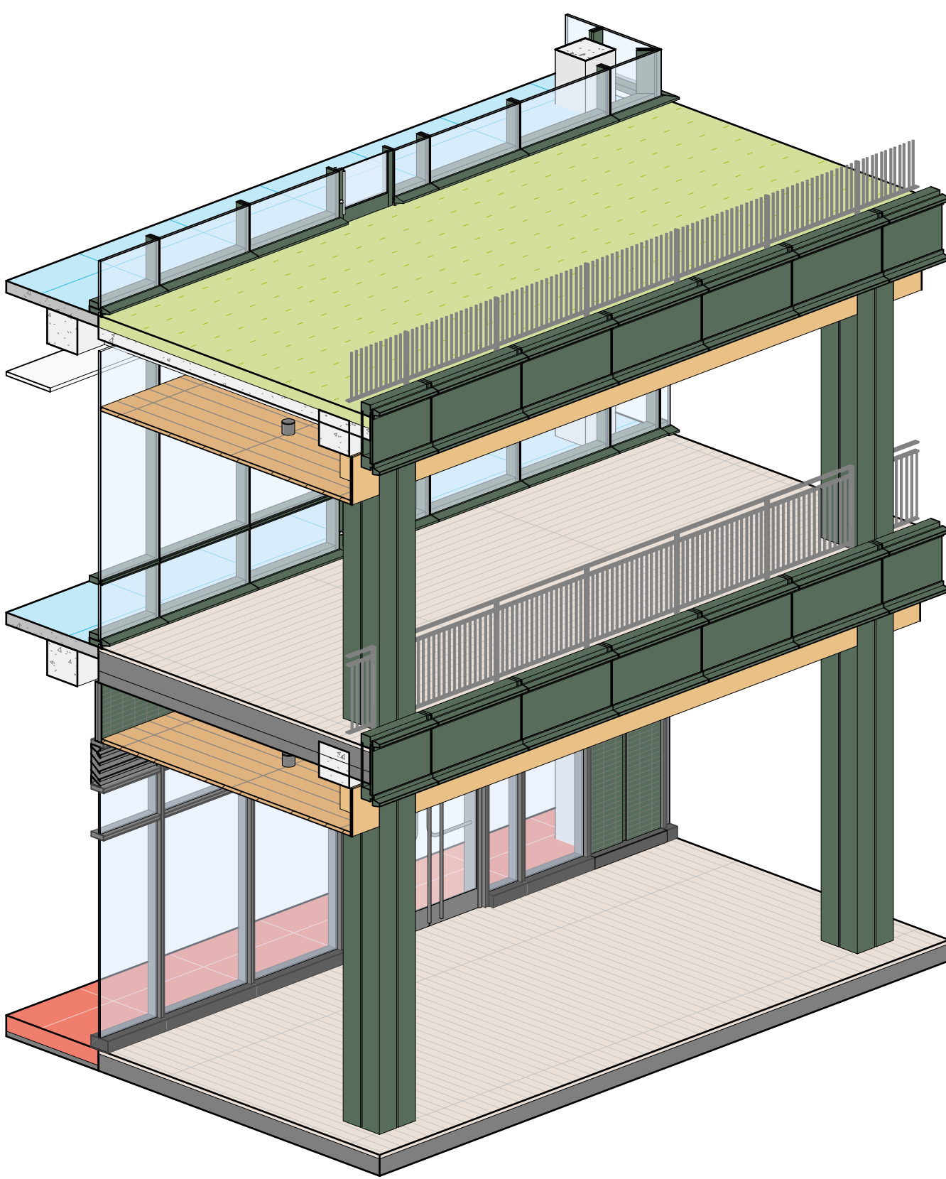
9 ENCLOSURE TYPE D2
